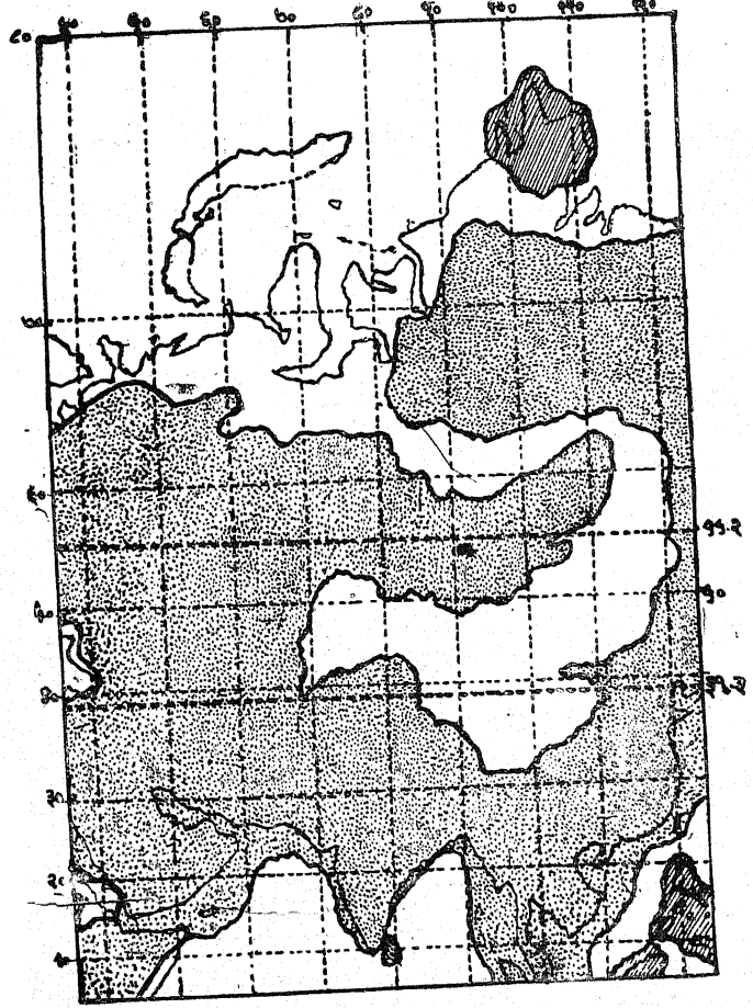
चित्र ५१-जंबू द्वीप दो लाख से अस्सी हजार बरस पहले तक ग्रंथकार की कृपा [ वेद-काल-निर्णय से ]
